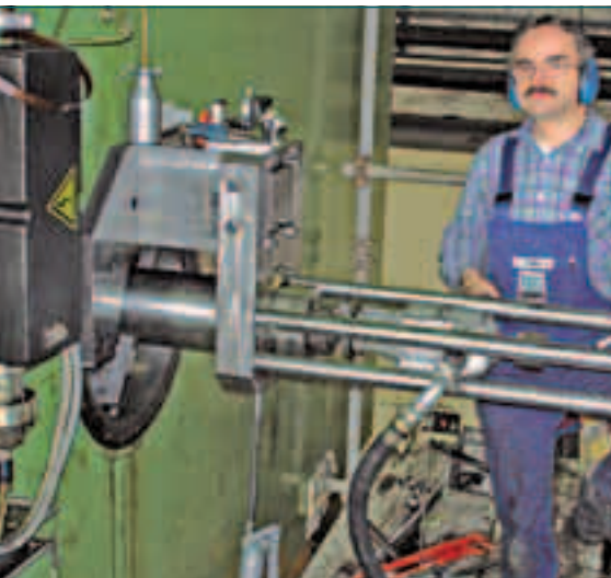
Justage der Ausspindelvorrichtung zur Pressengetriebebearbeitung.
